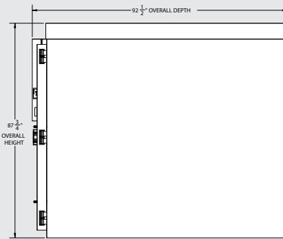
BF402DP-1P / BF402AP-1P
